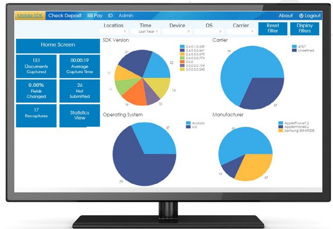
Abbildung 1. Kofax Mobile SDK-Dashboard-Ansichten
